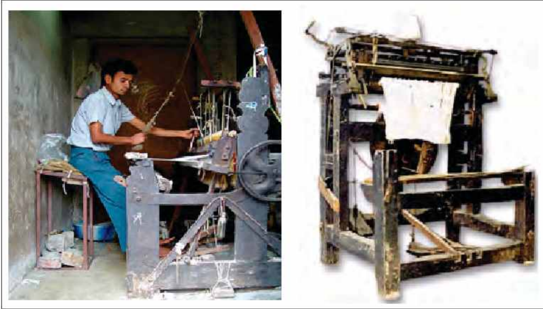
پیروں سے تانے کے تار اٹھانے والی کھڈی (Treadle Loom)
