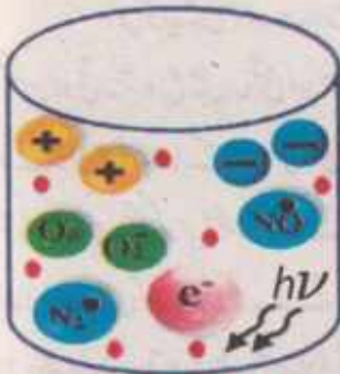
فصل 7.3(a) پلازما
