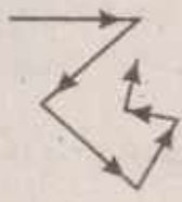
بے ترتیب راستہ شکل 2.7(a)
