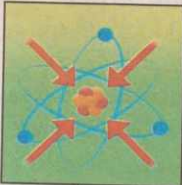
شکل 3.6 نیوکلینس
