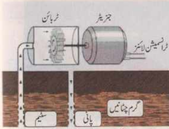
شکل 5.17 جیوتھرمل پلانٹ
