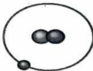
Deuterium ( {}^2_1\text{H} )
