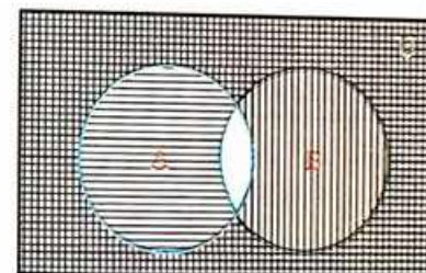
A' \cap B' (Fig. 2)
