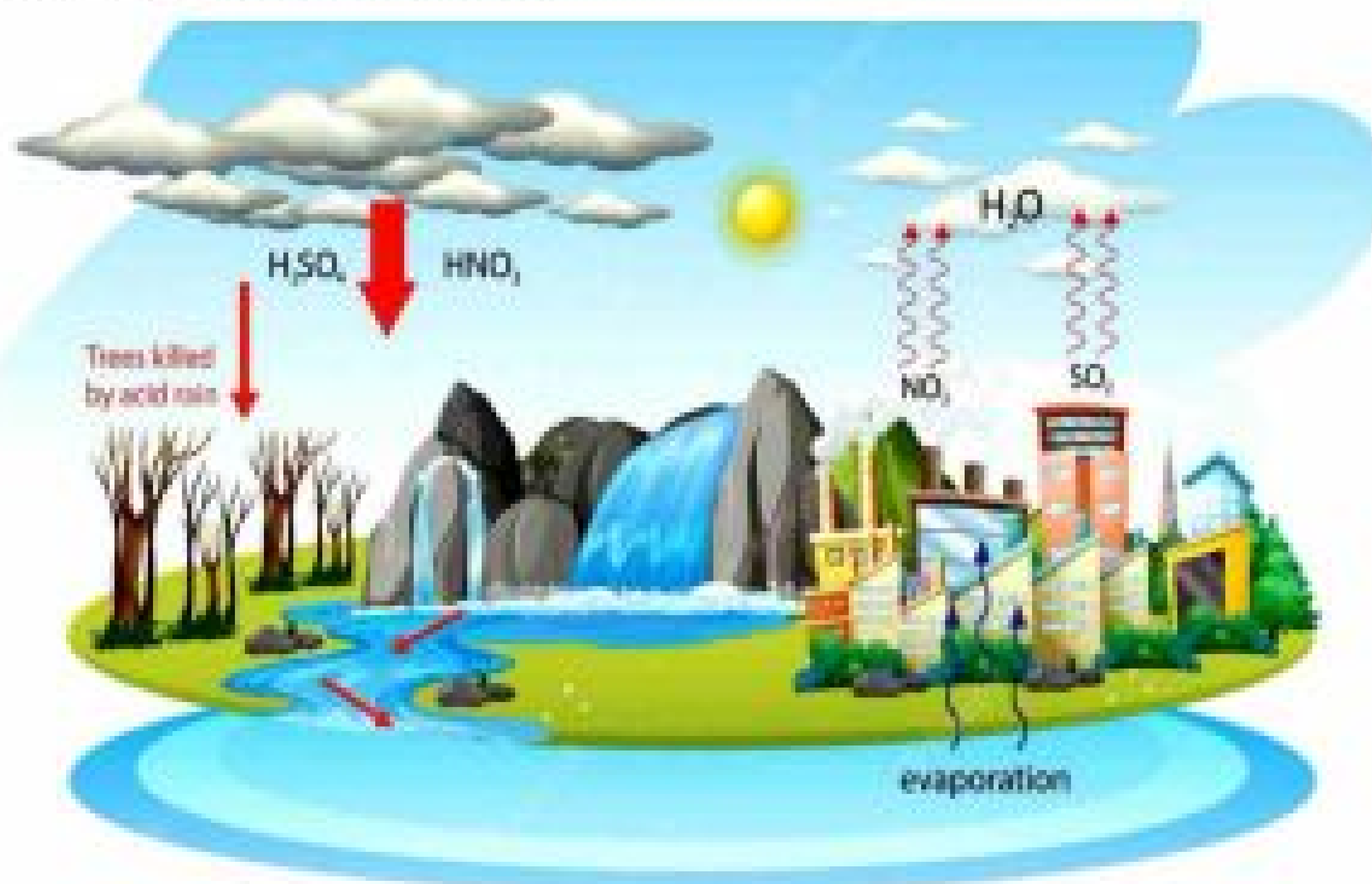
Fig. 25.10 Acid rain
