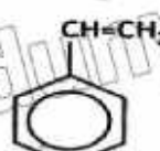
styrene
