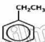
ethylbenzene
