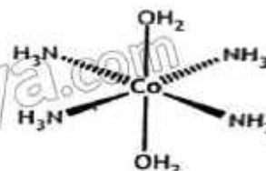
trans-tetraamminediaquacobalt(II)
