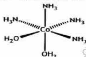
cis-tetraamminediaquacobalt(II)
