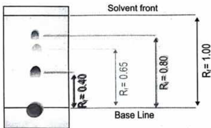
Fig 19.7 R_f Value
