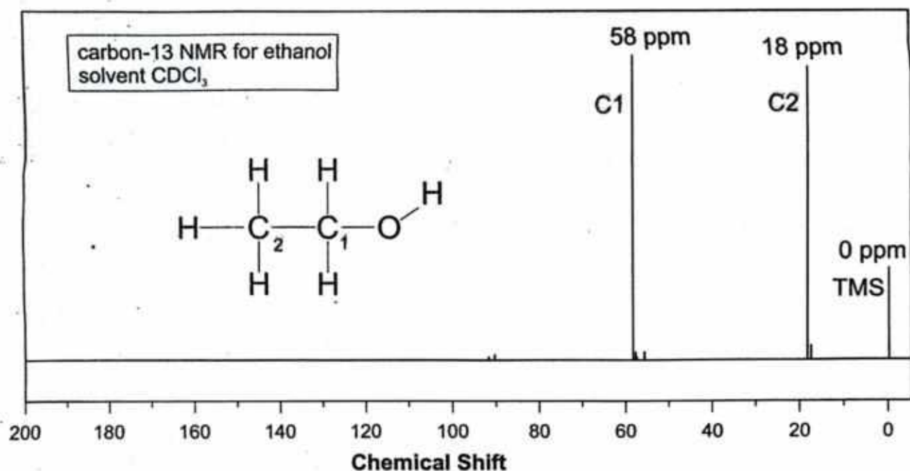
Fig 18.10: ^{13}\text{C} -NMR of ethanol
