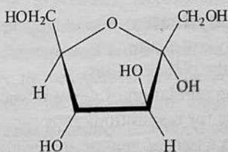
\alpha -D-fructose
