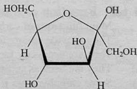
\beta -D-fructose
