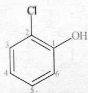
2-Chlorophenol ( o -Chlorophenol)
