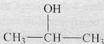
2-Propanol
