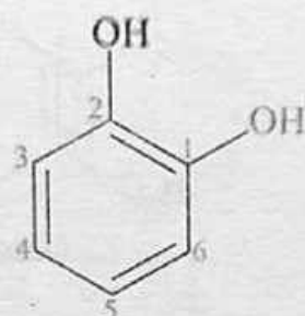
1,2-Benzenediol (Catechol)
