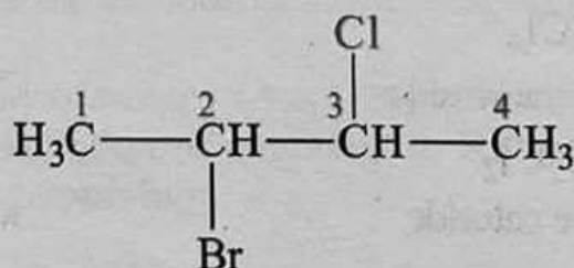
2-Bromo-3-chlorobutane
