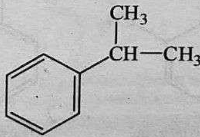
Cumene
