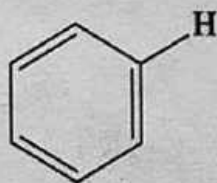
Benzene
