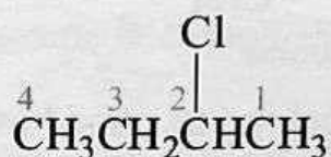
2-Chlorobutane
