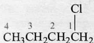
1-Chlorobutane
