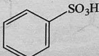
Benzenesulphonic acid
