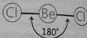
VSEPR model of \text{BeCl}_2
