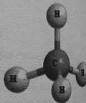
VSEPR Model of \text{CH}_4
