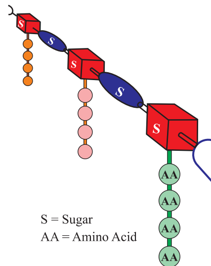
Fig: 6.2 Peptidoglycan
