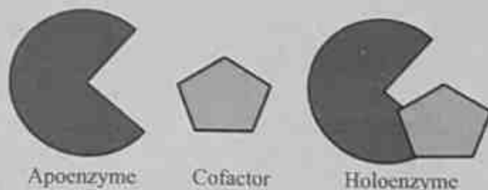
Fig.3.2 Holoenzyme
