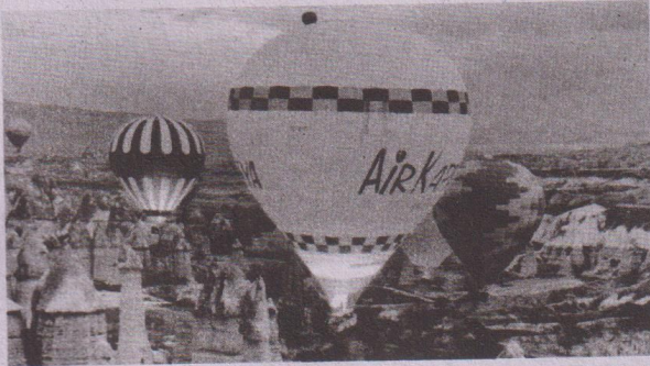
شکل 6 گرم ہوا والے غبارے کے ٹمپرچر بڑھنے سے ہوا کی انٹرل انرجی بڑھتی ہے۔
