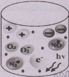
شکل 3 پلازما
